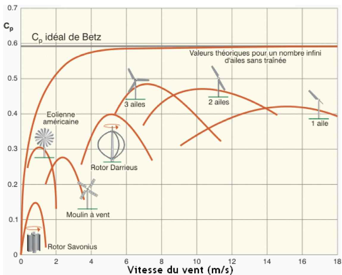
Figure 6 : efficacité des types d'éolienne en fonction de la vitesse du vent.
