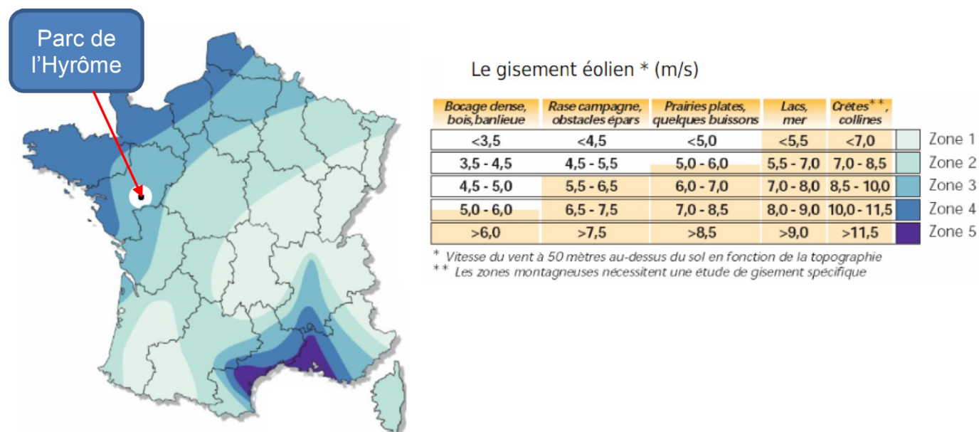
Figure 5 : carte du potentiel du vent en France métropolitaine.
